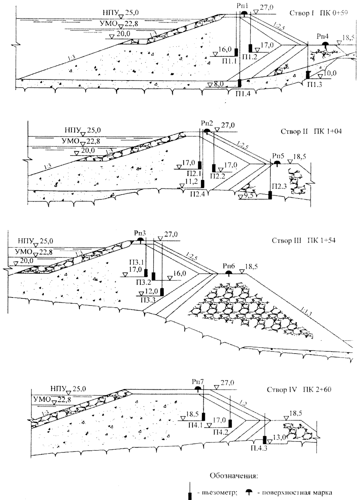
Рис. П.7.2. Схема расположения КИА в створах I-IV земляной плотины
