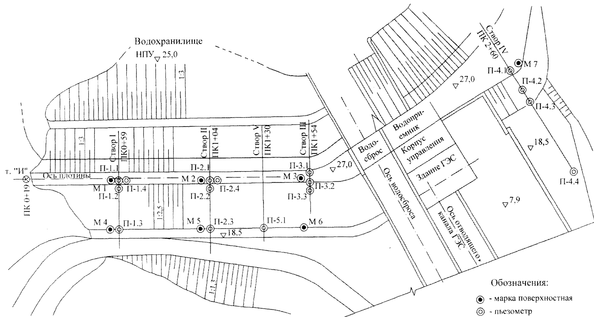
Рис. П.7.1. Схема расположения контрольно-измерительной аппаратуры на земляной плотине (план)
