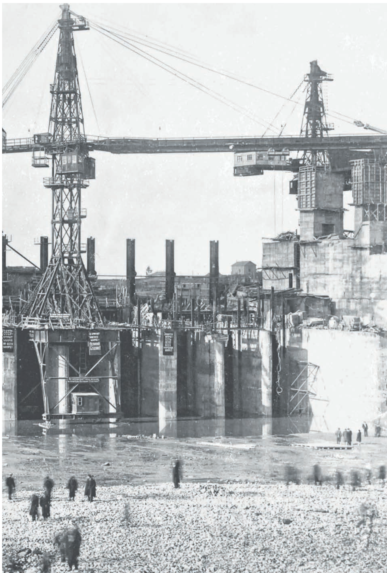
Строительство Верхне-Сайфской ГЭС, 50-ые годы
